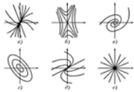
1. Особые точки линейной автономной системы на плоскости
